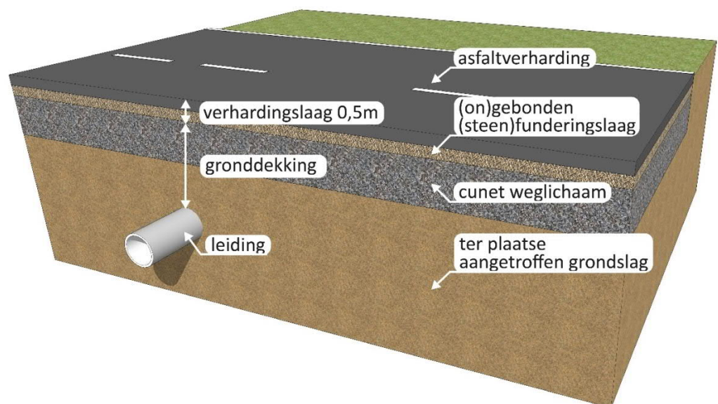
Figuur 5.4: schematische weergave van de gronddekking bij Open Ontgraving
