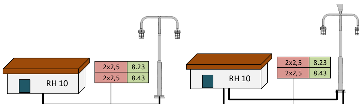
Afbeelding 13: Kabel tussen relaishuis en waarschuwingsinstallatie bij dienstoverpad (wido) zonder en met bel.
