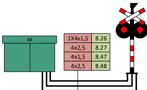
Afbeelding 64: kabels tussen S&amp;B schakelkast en S&amp;B RGP met 2 lampen en bel
