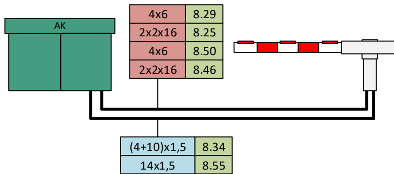
Afbeelding 62: kabels tussen S&amp;B schakelkast en S&amp;B overwegsteller HSM10E
