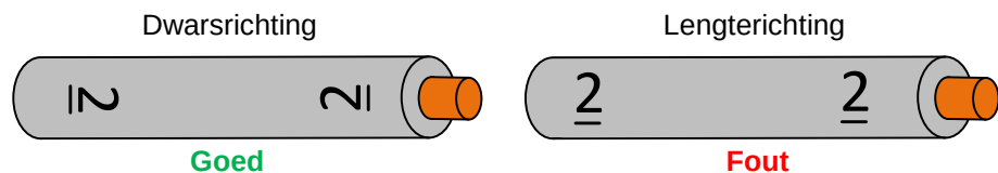
Afbeelding 86: richting van adermarkering op adermantel
