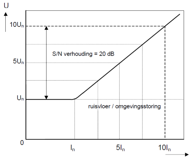
Afbeelding 96: Lineair verband meetpunten en bepaling signaal / stoorverhouding
