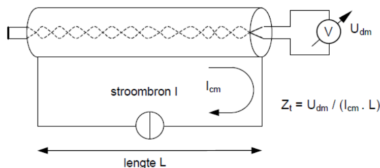
Afbeelding 94: principeschema transfer impedantie meting
