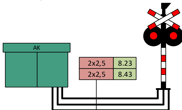
Afbeelding 62: kabels tussen S&amp;B schakelkast en S&amp;B overwegsteller HSM10E
