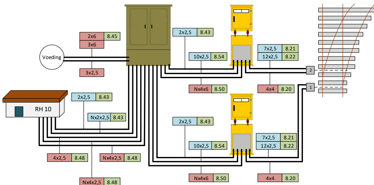
Afbeelding 45: Kabel bij wisselaansturing met wisselverdeelkast. Voeding kan zowel vanaf relaishuis als voedingskast.
