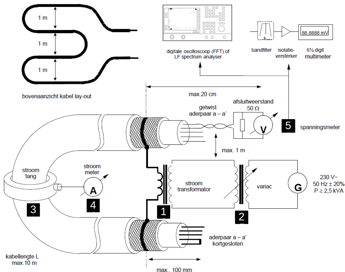
Afbeelding 95: Meetopstelling symmetrische transfer impedantie meting
