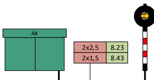
Afbeelding 65: kabels tussen S&amp;B schakelkast en AG
