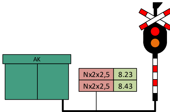
Afbeelding 74: kabels tussen S&amp;B schakelkast en verkeerslicht (h)ali
