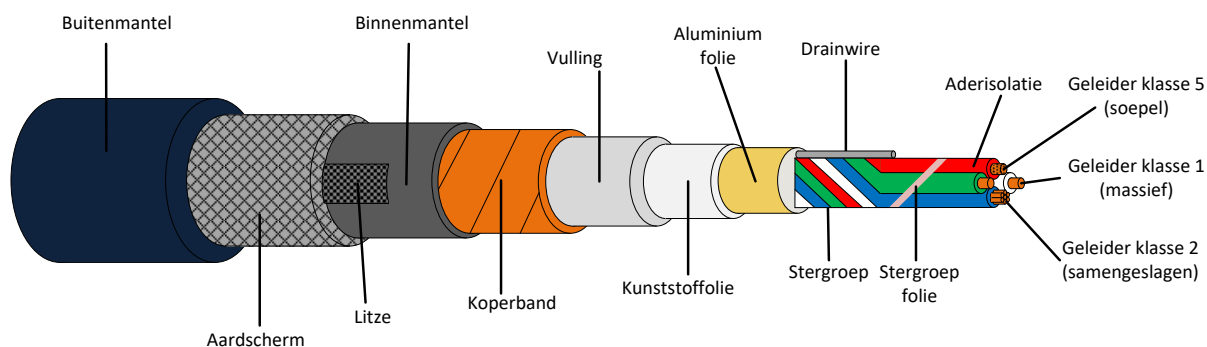
Afbeelding 92: kabelopbouw
