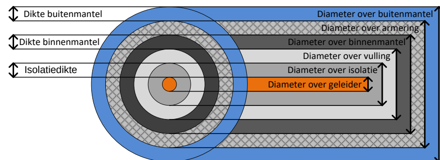
Afbeelding 93: maatvoering
