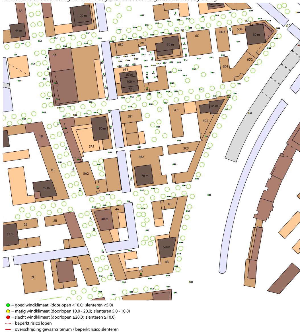
f3.7 Hinderkans en beoordeling windklimaat geplande bebouwingssituatie met begroeiing
