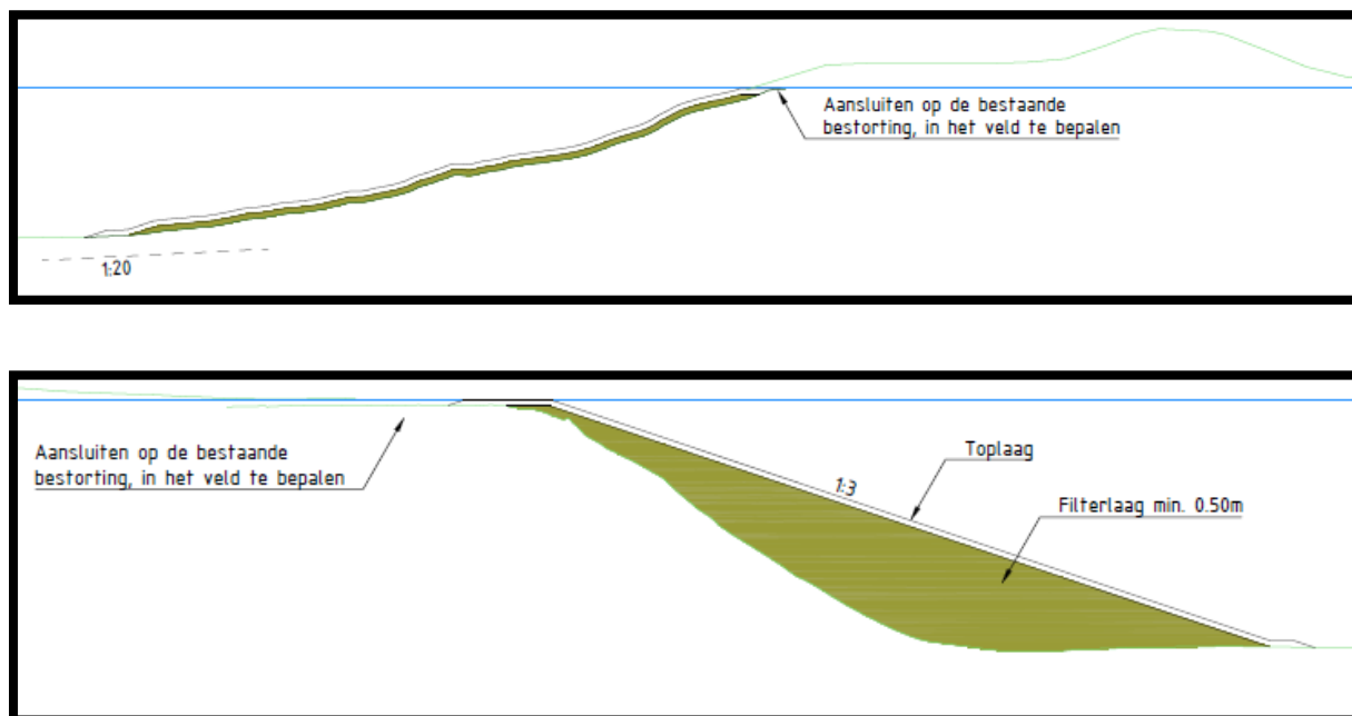
Figuur 3-1 Kenmerkende profielen
