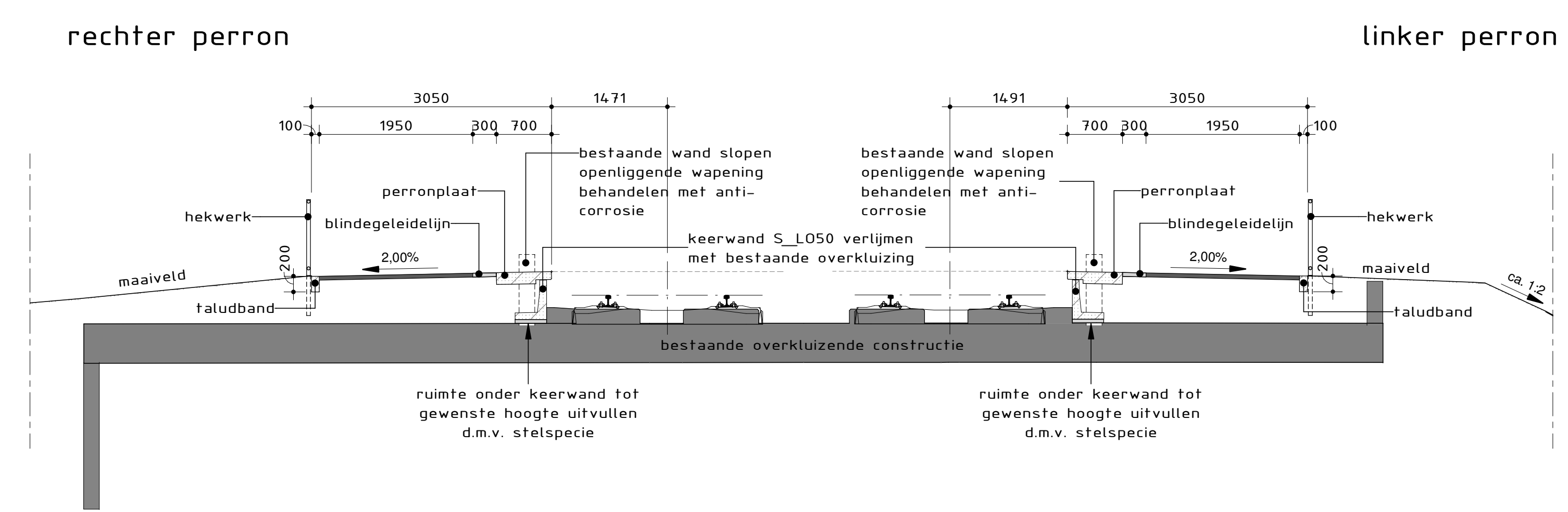
Dwarsdoorsnede A Schaal 1 : 50
