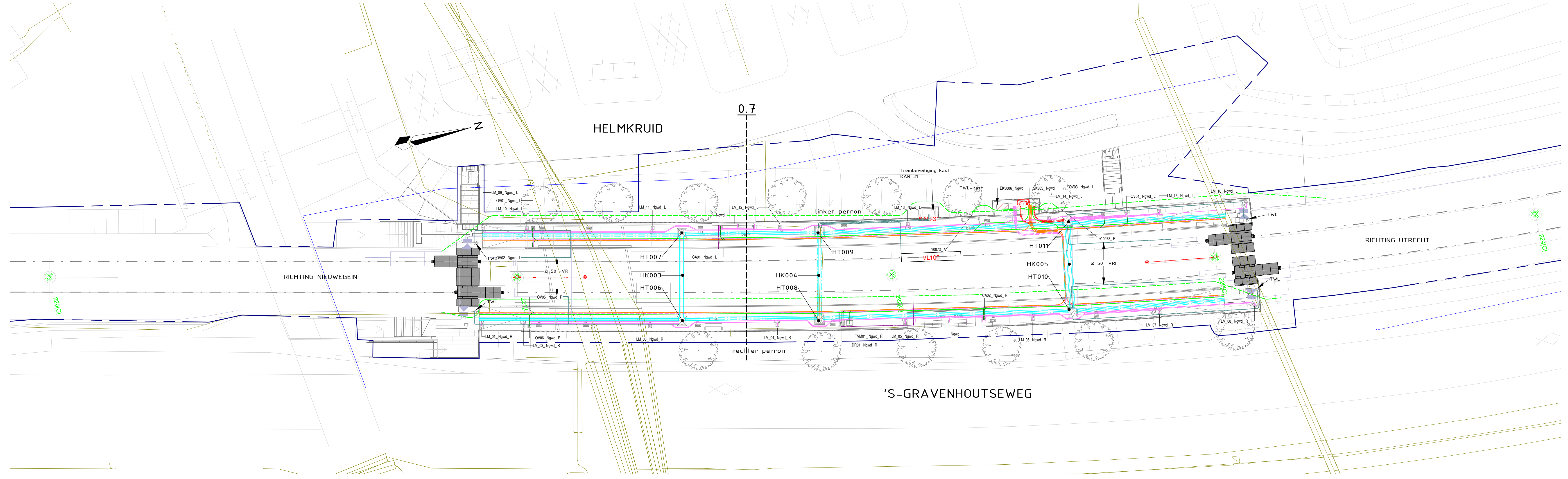
Bovenaanzicht ondergrondse infra Schaal 1 : 200
