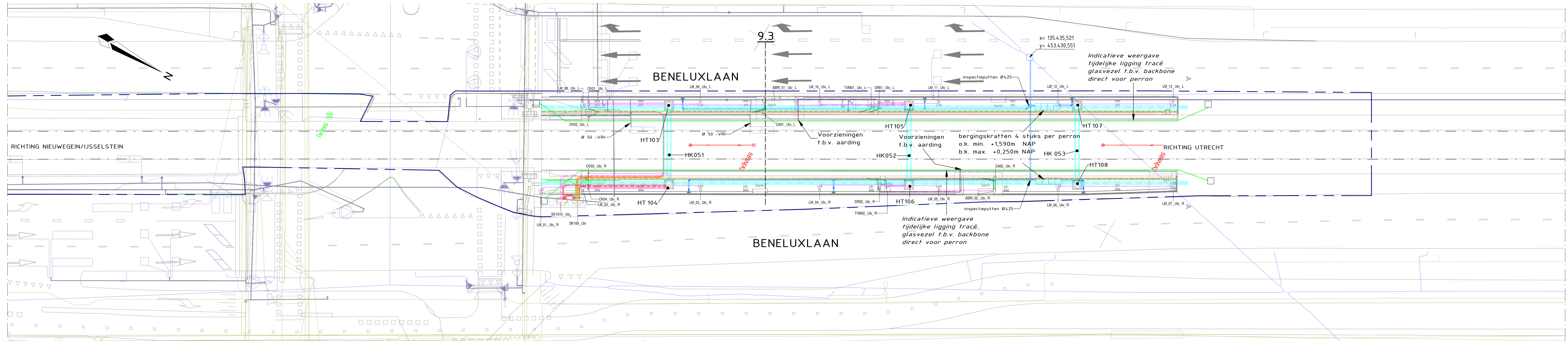
Bovenaanzicht ondergrondse infra Schaal 1 : 200
