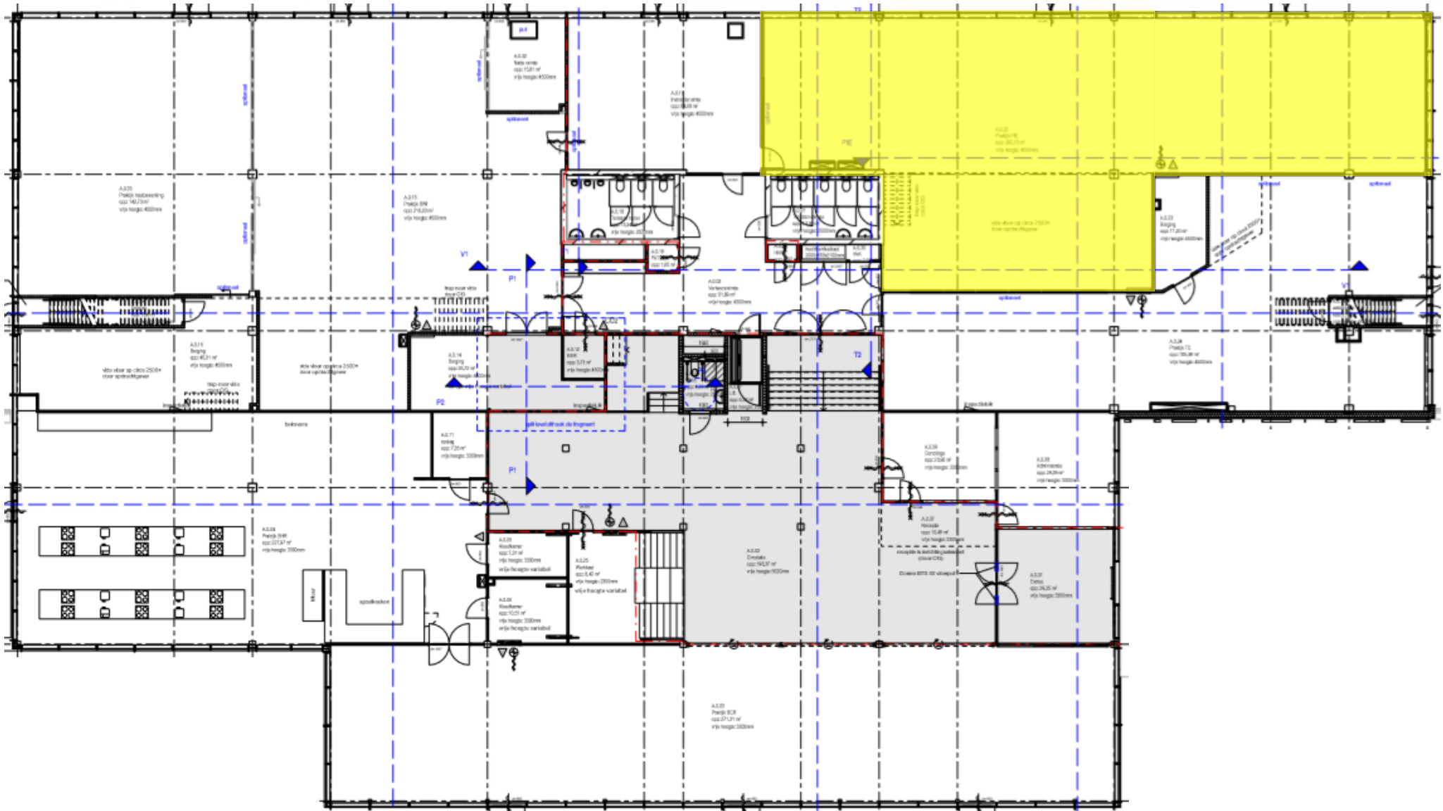
Begane grondvloer
