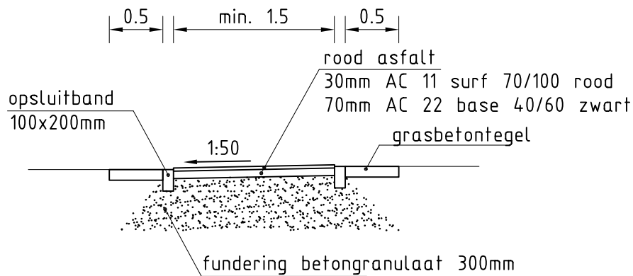
FIETSPAD 1 RICHTING DOORSNEDE
