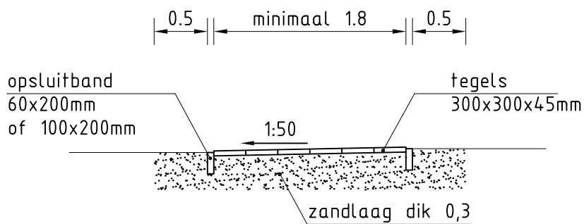
VOETPAD DOORSNEDE
