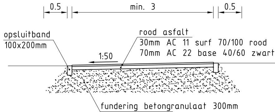
FIETSPAD 2 RICHTINGEN DOORSNEDE
