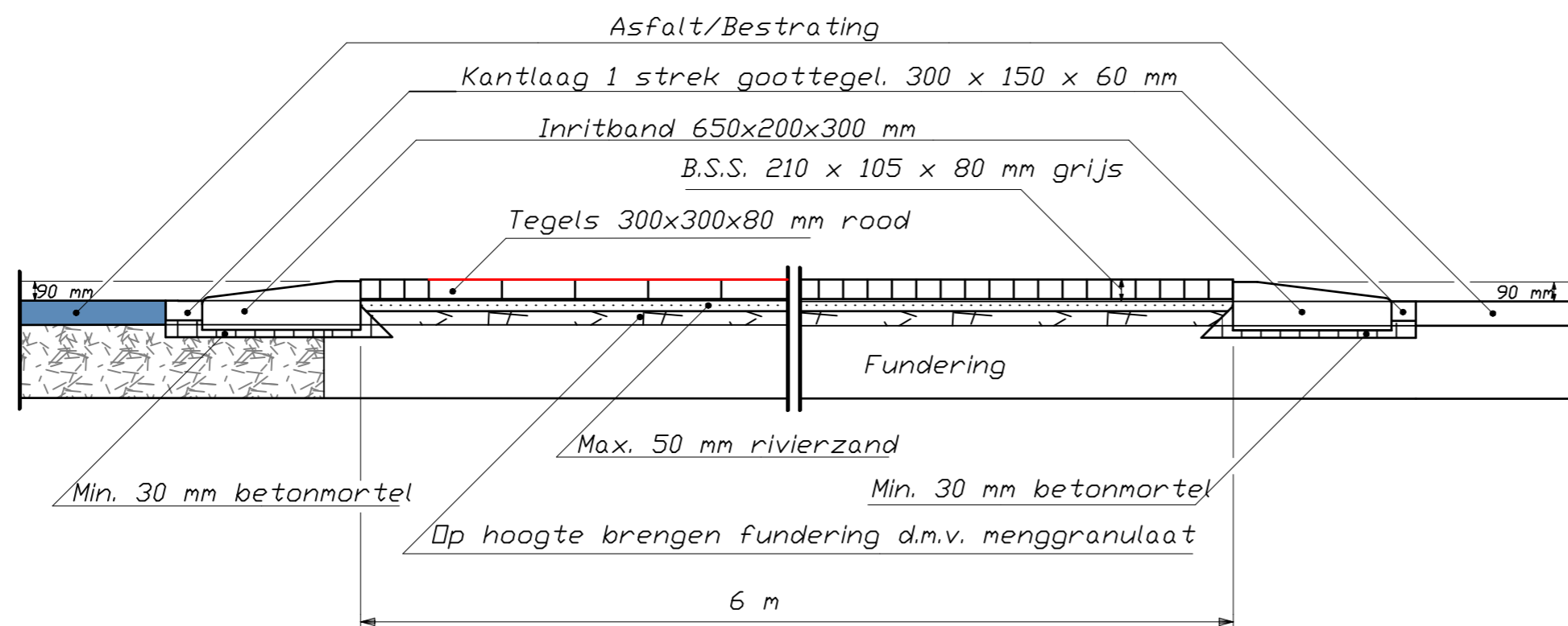
Doorsnede A-A
