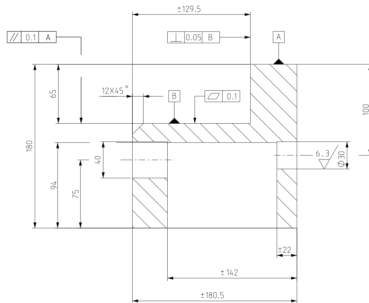
DOORSNED E E-E SCHAAL 1:2,5
