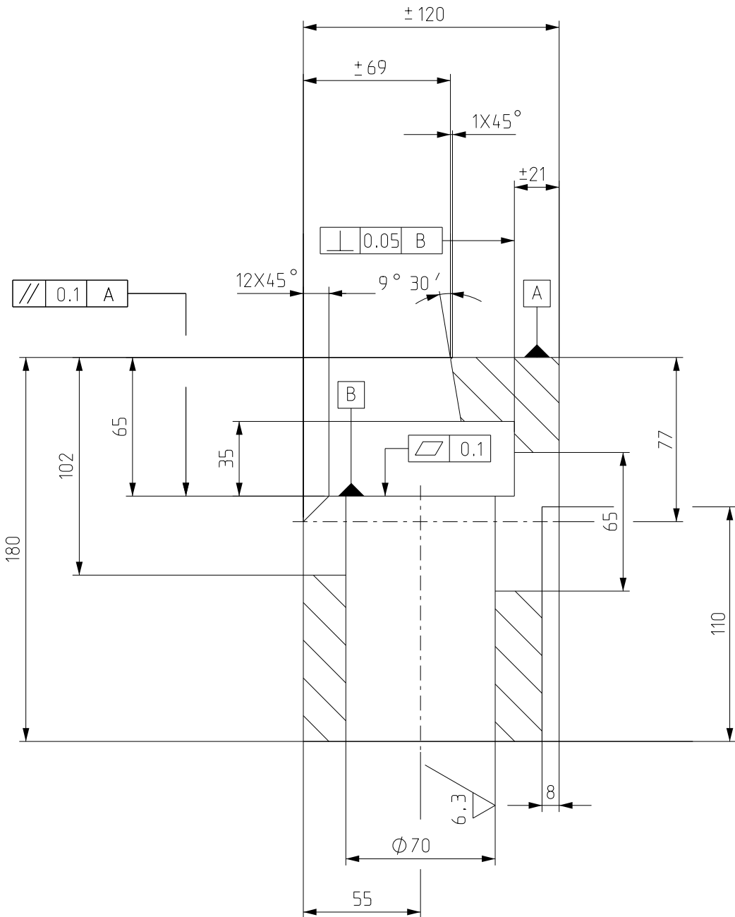
DOORSNED E B-B SCHAAL 1:2,5
