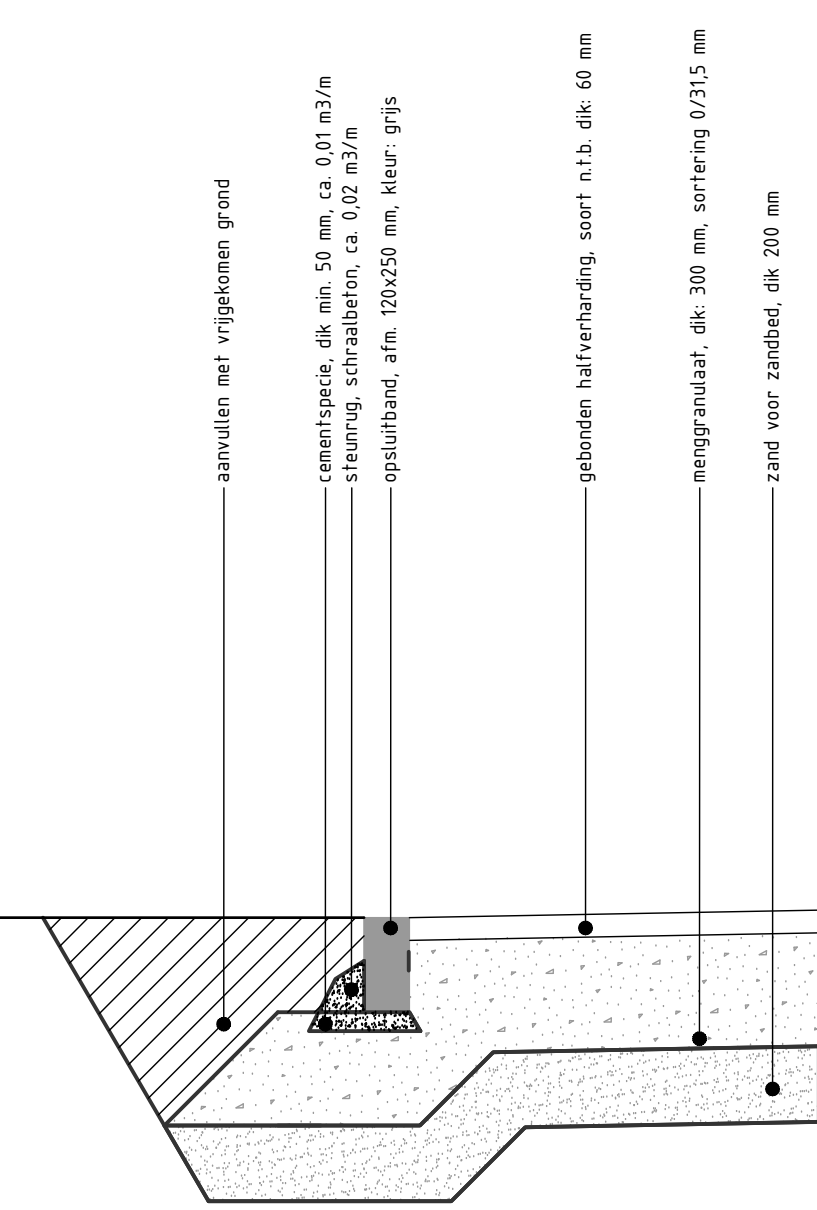
Principedetail kantopsluiting d.m.v. opsluitband op puinfundering (halfverharding) schaal 120
