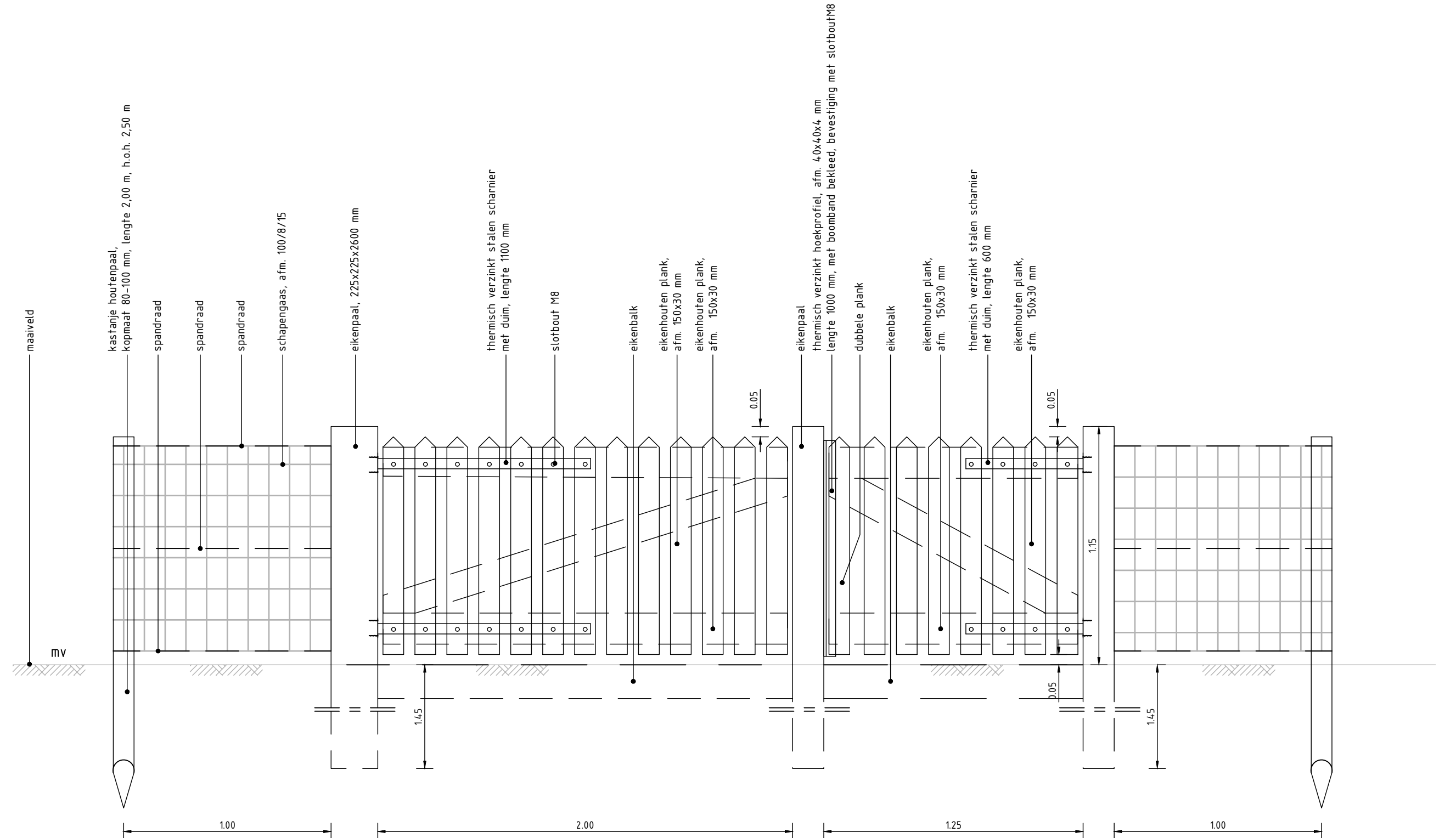
Principedetail poort met klaphek voor voetgangers schaal 120
