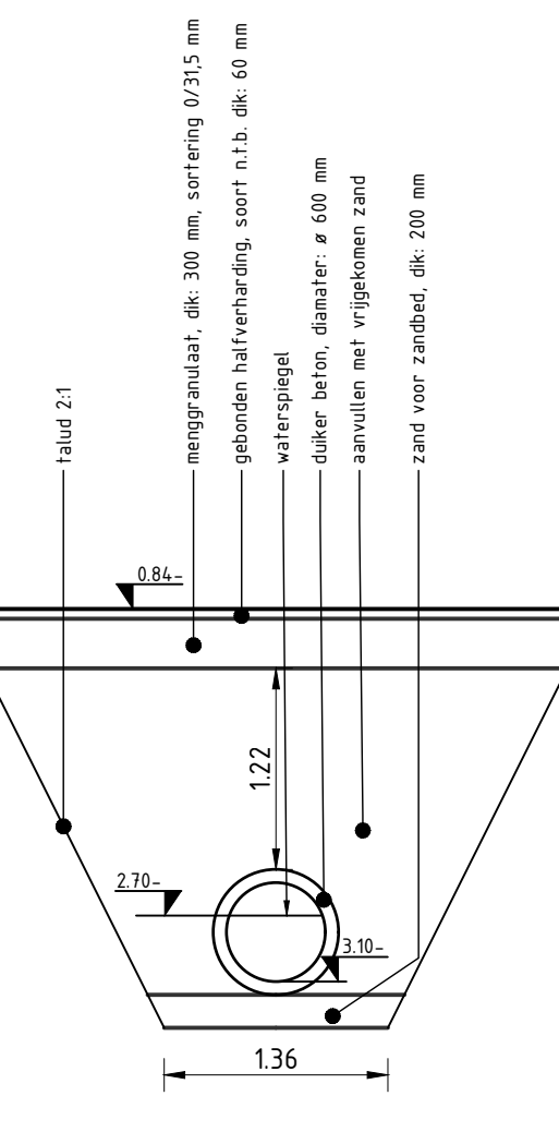
Principedetail doorsnede duiker schaal 150
