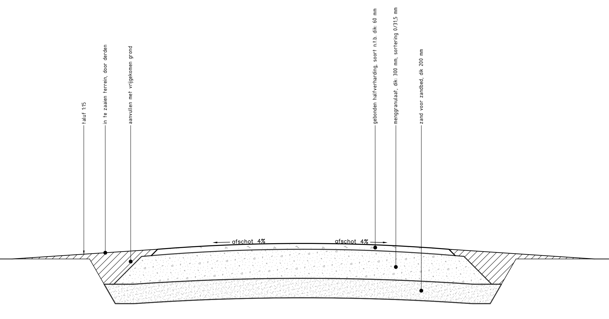
Principedetail halfverharding op puinfundering en zand schaal 120
