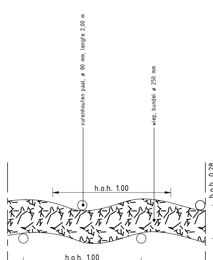
Principedetail wiepen schaal 120
