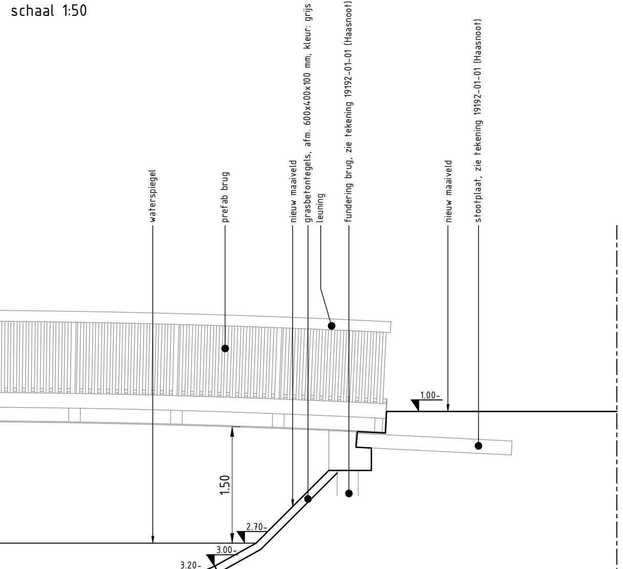
Detail C-C brug schaal 150
