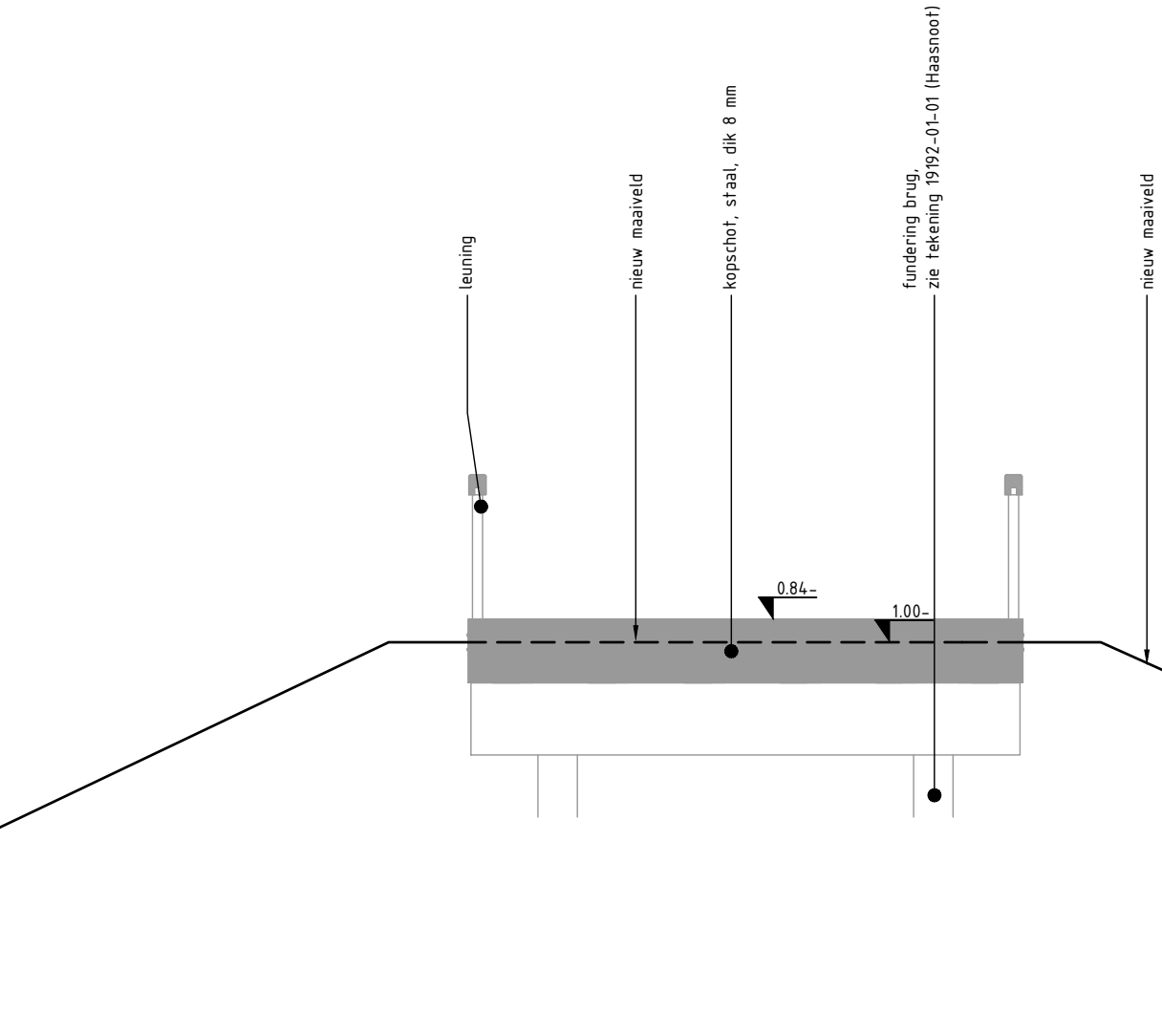
Detail D-D brug schaal 150
