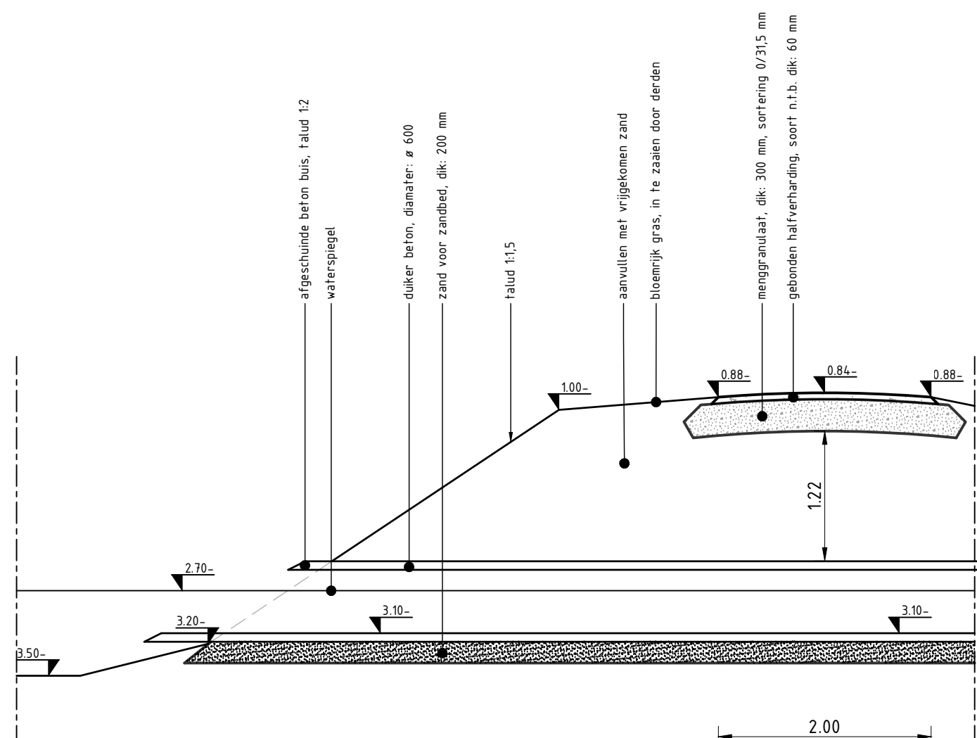
Principedetail doorsnede duiker schaal 150
