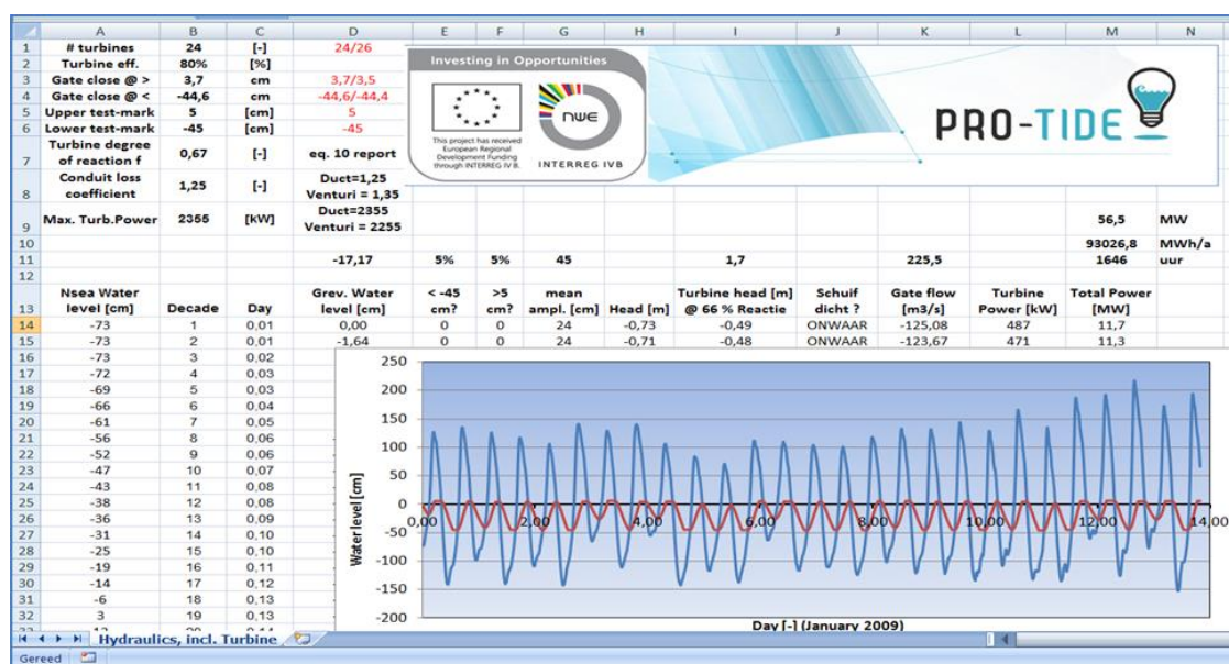
Figuur 8: Screen-shot van het hydro-energetisch model (Microsoft Excel)
