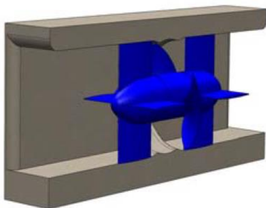
Figuur 7: Voorbeeld van turbine in rechthoekige doorlaat
