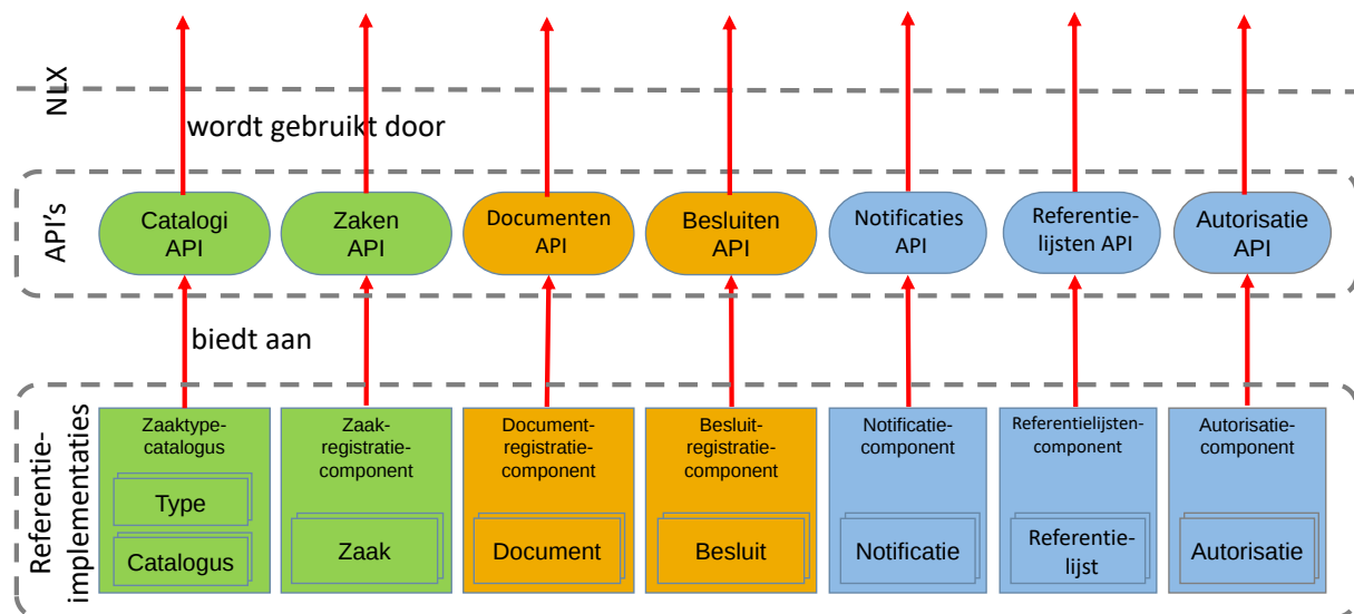
Figuur 1 Overzicht van ZGW API's en registraties
