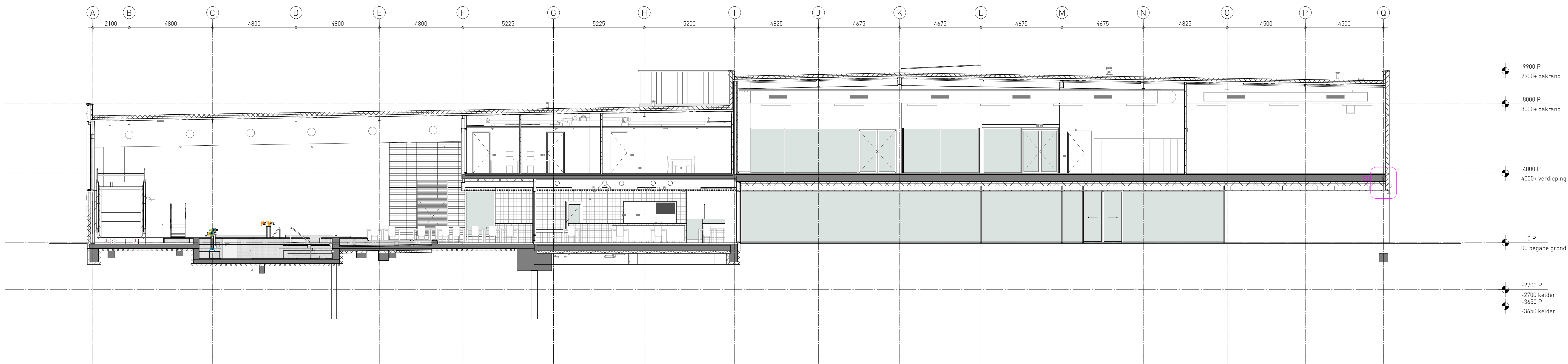
doorsnede A
