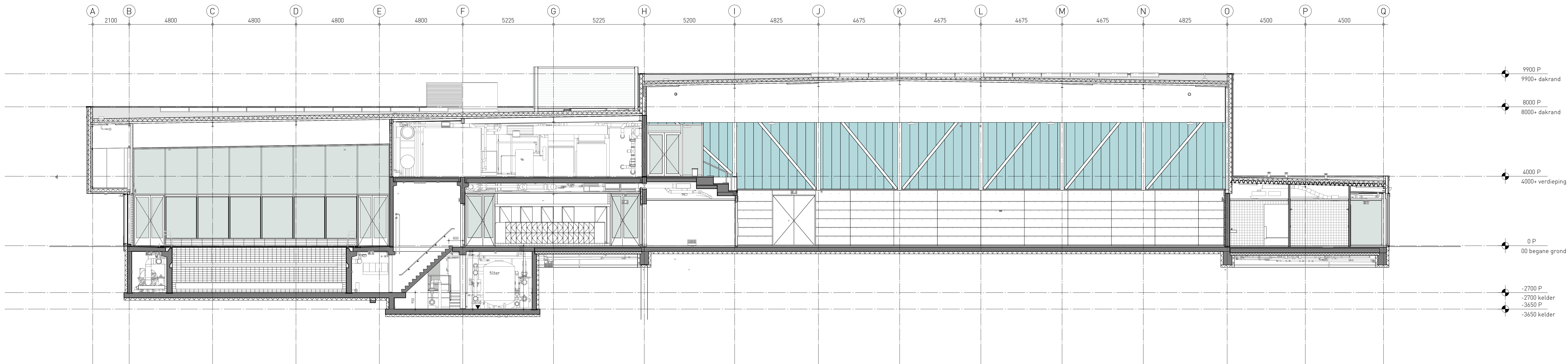
doorsnede B
