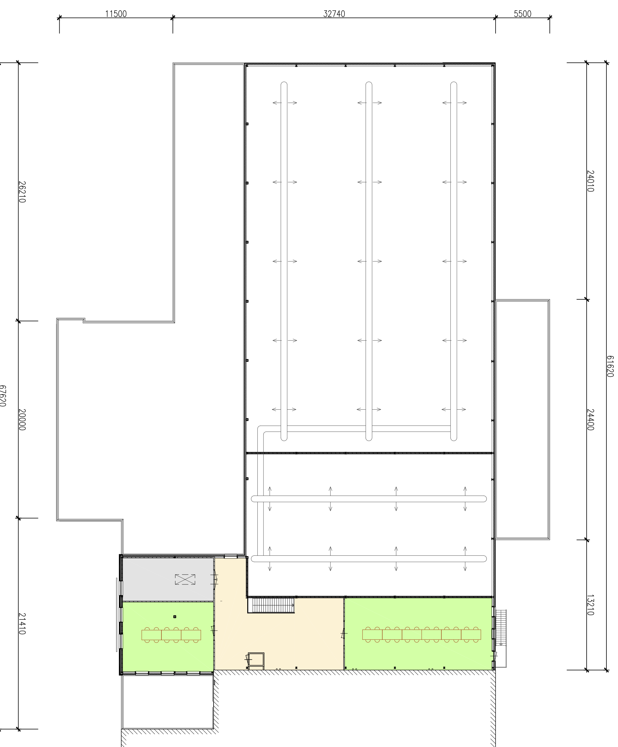
PLATTEGROND VERDERPING
