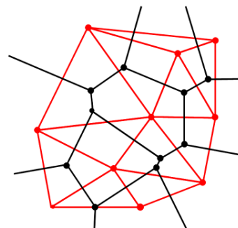
Figuur 1: Samenhang tussen Voronoi-polygoon (zwart) en Delauney-triangulatie (rood).
