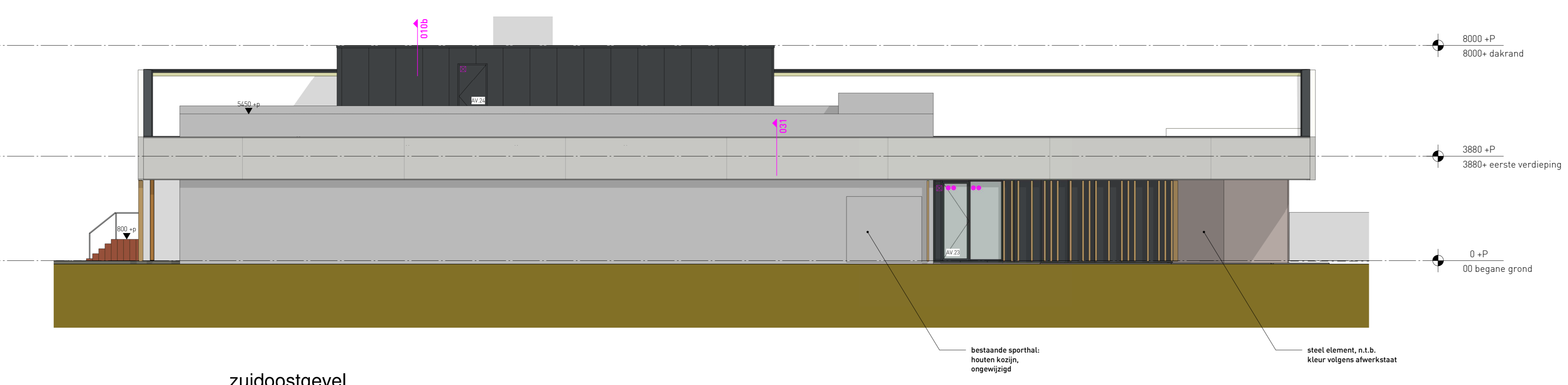
zuidoostgevel
