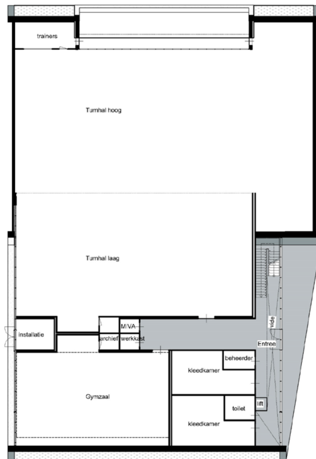
begane grond
