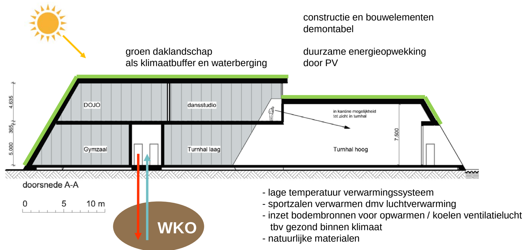
doorsnede
