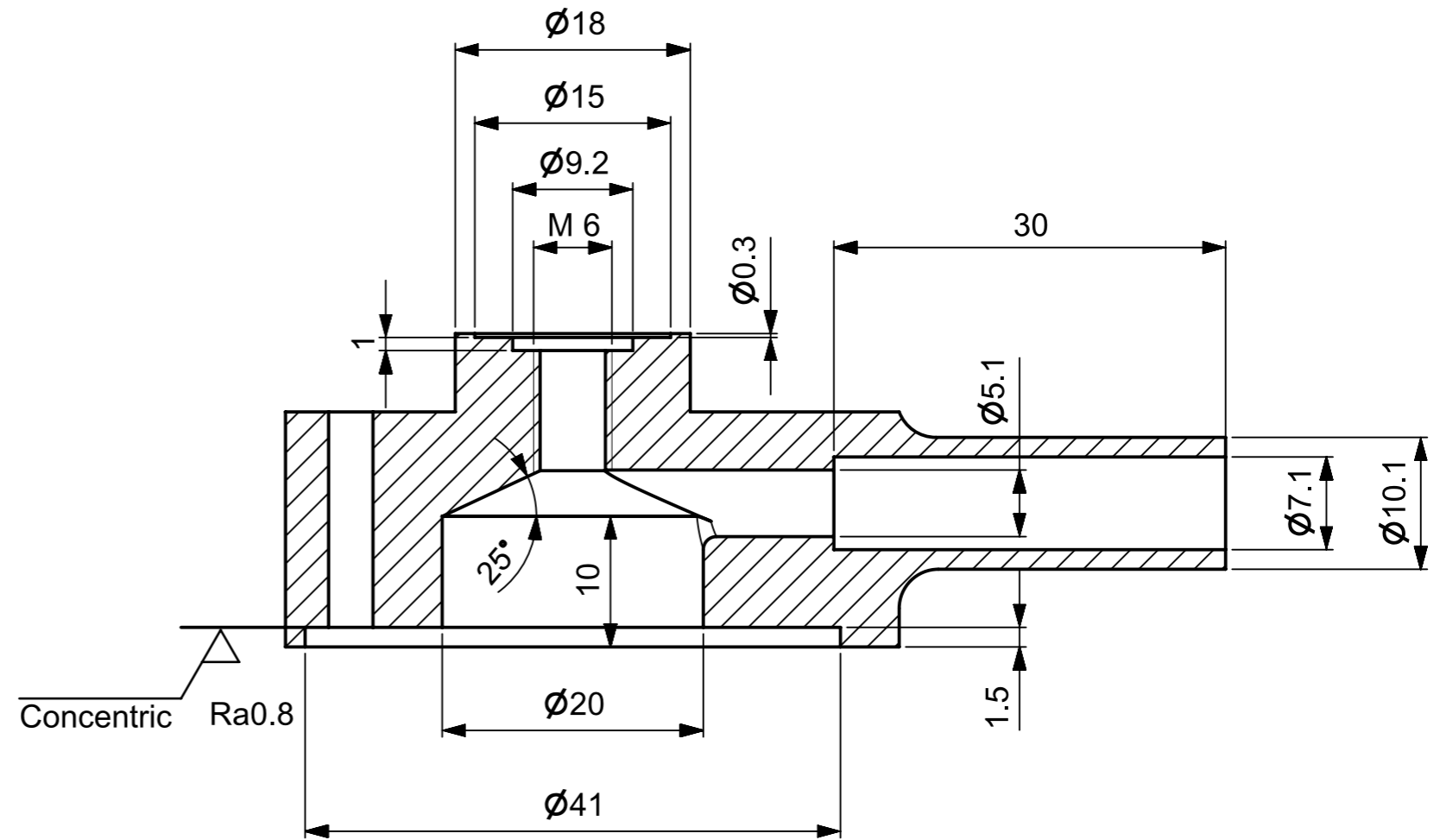
SECTION A-A
