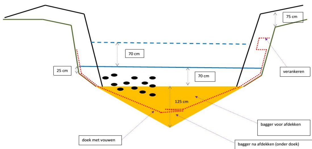
Principeschets Project Tankval door afdekken met 0,75 meter schone grond (bron: Natuurmonumenten)
