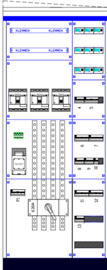
Verdeelkast HKL hxbxd 2000x800x450mm Systeemkast uit plaatstaal IP 54
