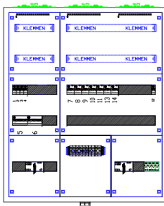
Verdeelkast OVK-2.2 Wandkast uit plaatstaal IP 41 hxbxd 800x950x210mm
