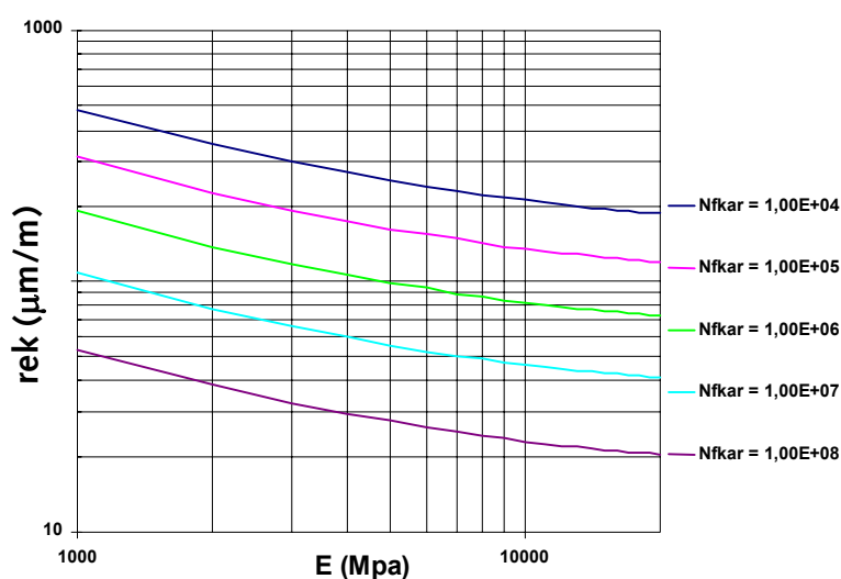
Figuur 5.4 Karakteristieke vermoeiingsrelatie asfalt
